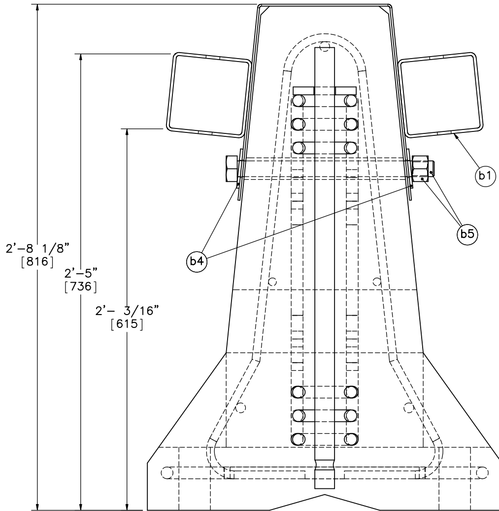
SECTION A-A
