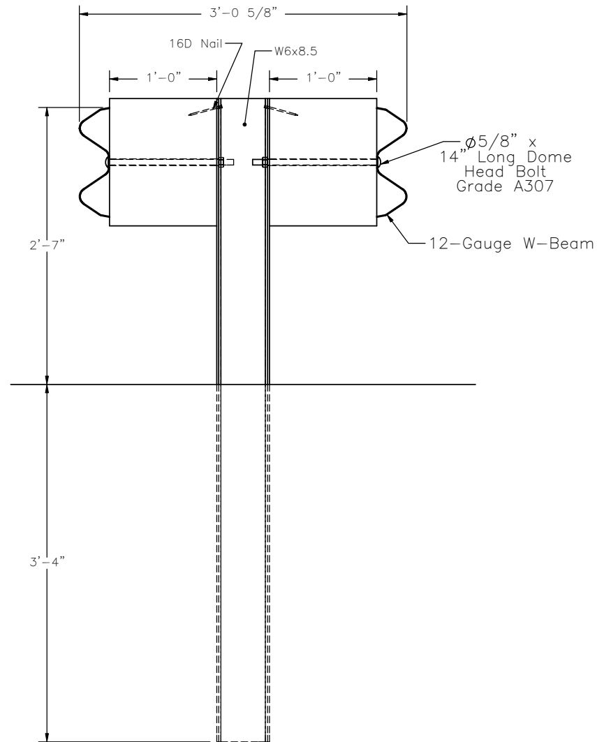
SECTION A-A
