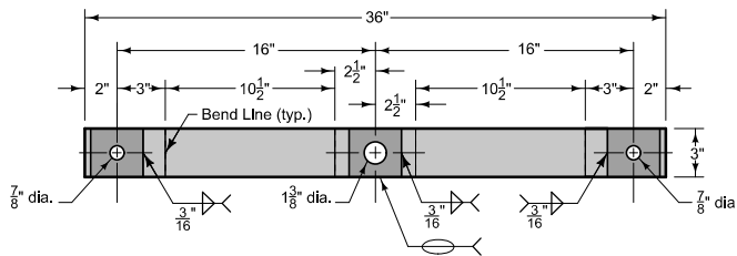
TIE-DOWN STRAP (before bending)
